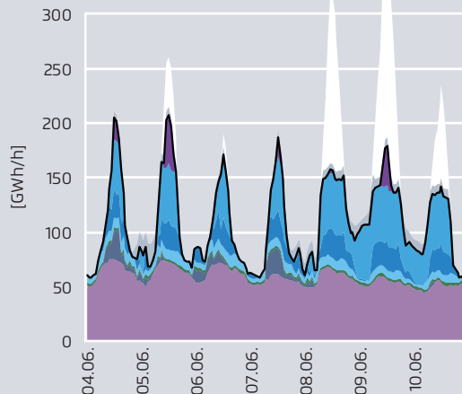
Nachfrage Sommerwoche
