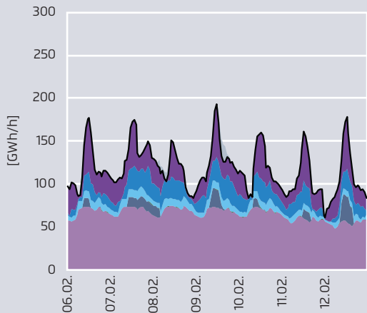
Nachfrage Winterwoche
